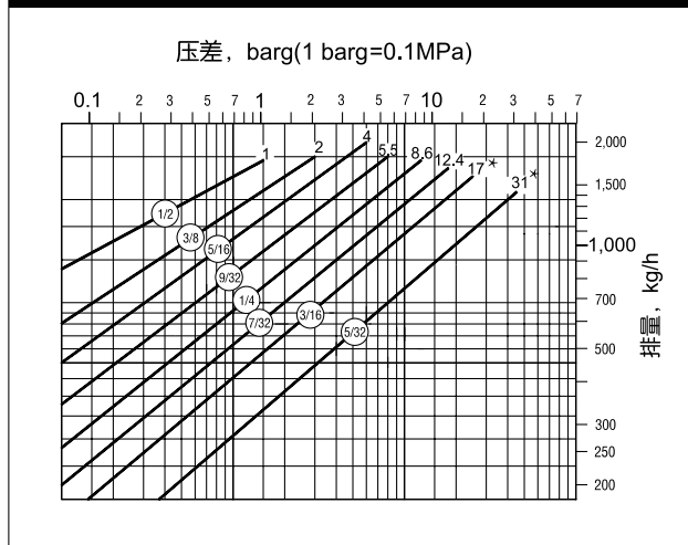
995F 排量图
