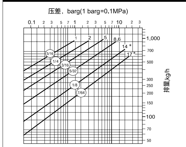
994F 排量图
