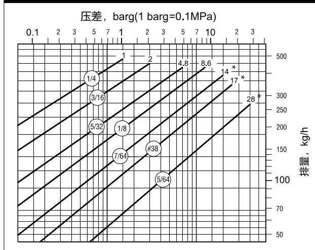
993F 排量图
