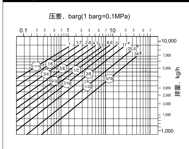
996F 排量图
